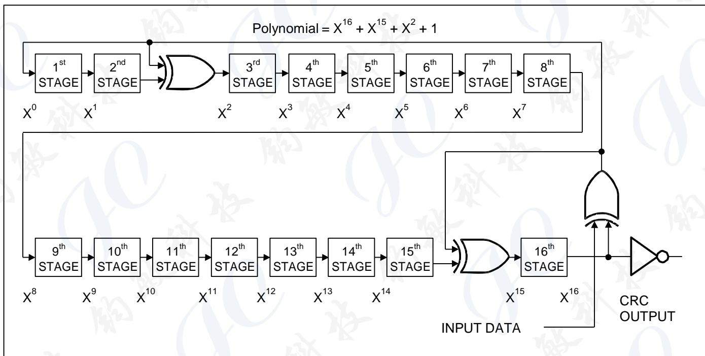
图 13. CRC-16 硬件说明及多项式
