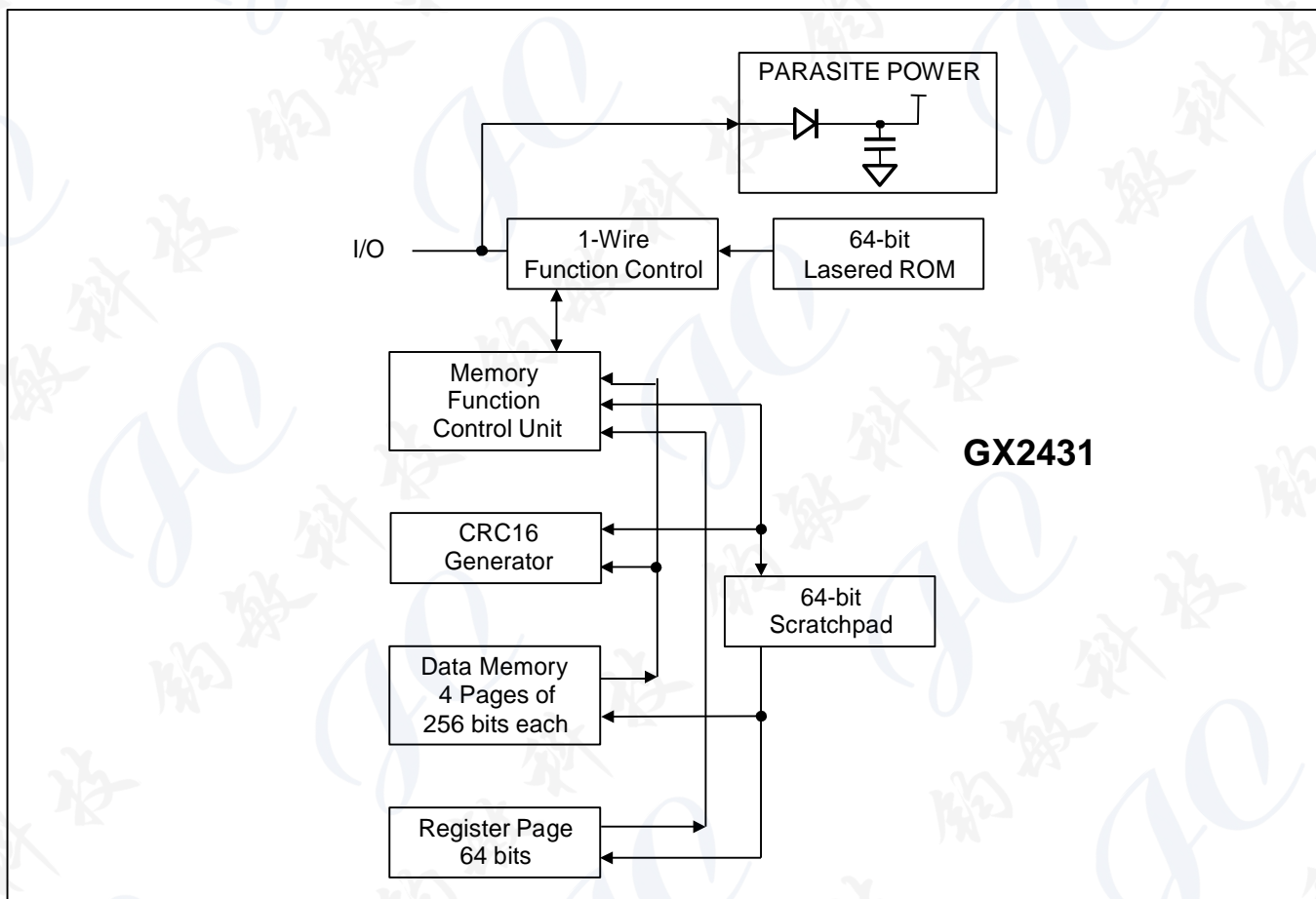
图 1. 结构框图
