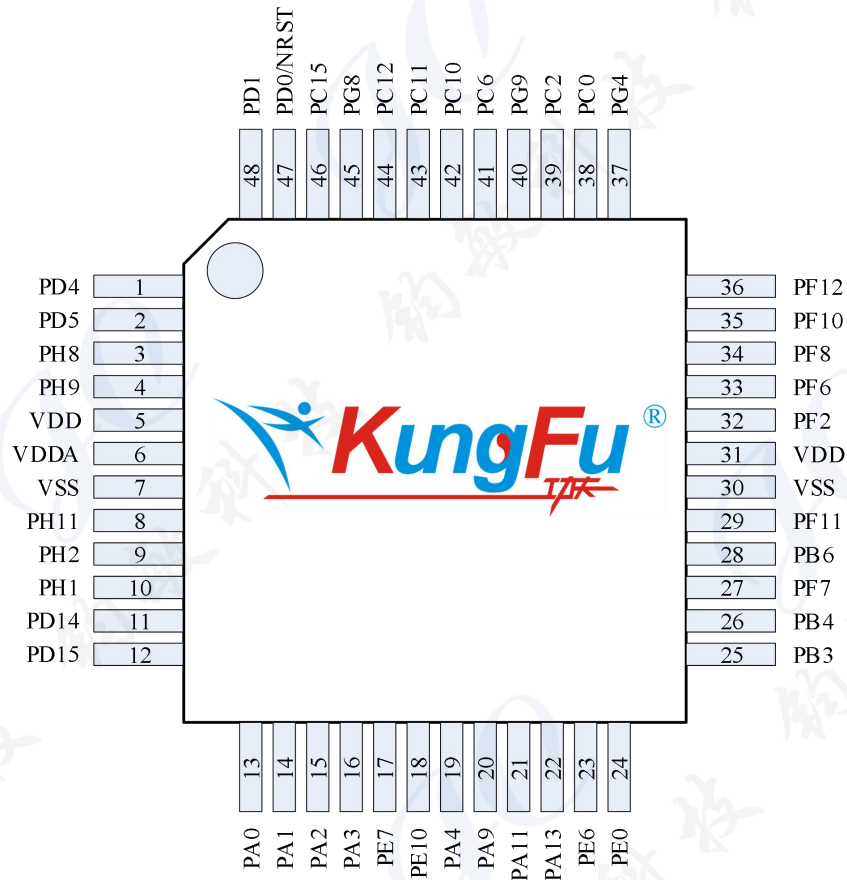
图 2-4 LQFP48
