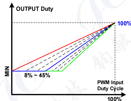
图 3 转速斜率与最低转组合
