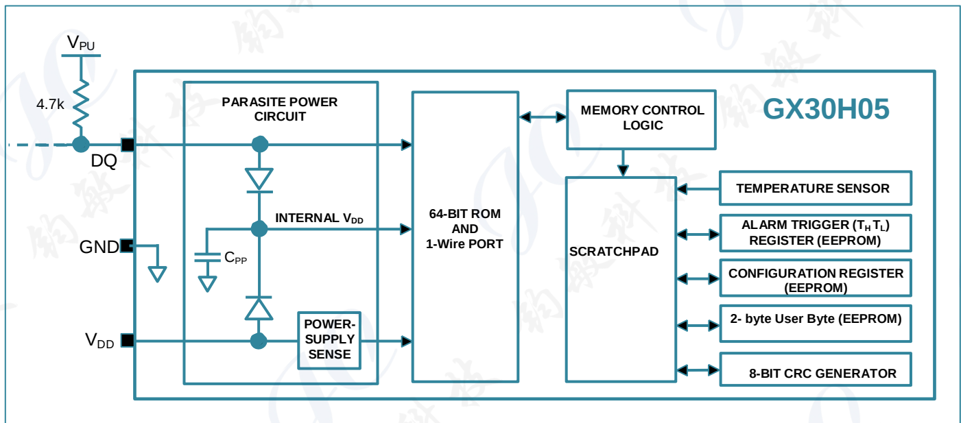
图 1. GX30H05 的结构框图
