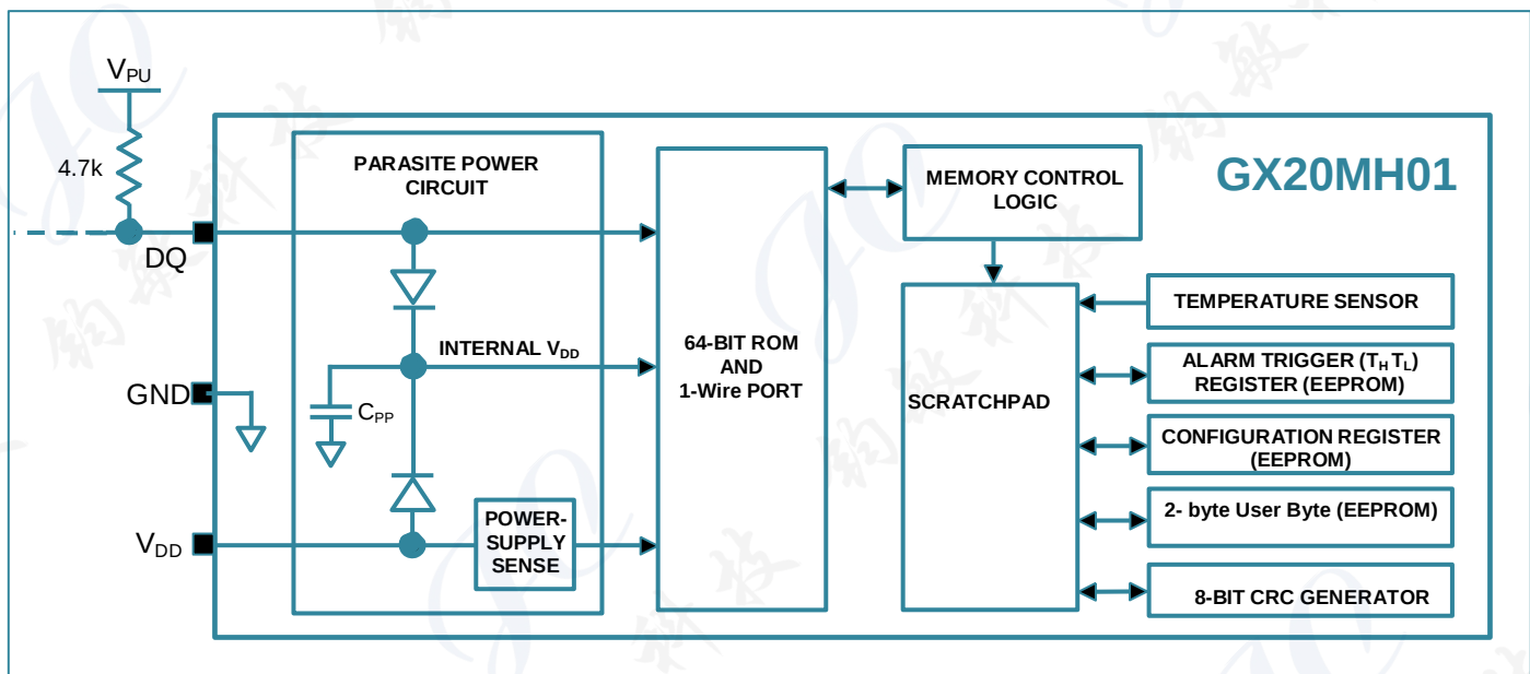
图 1. GX20MH01 的结构框图
