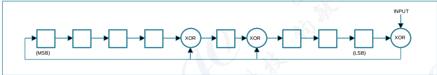
图 9. CRC 产生器
