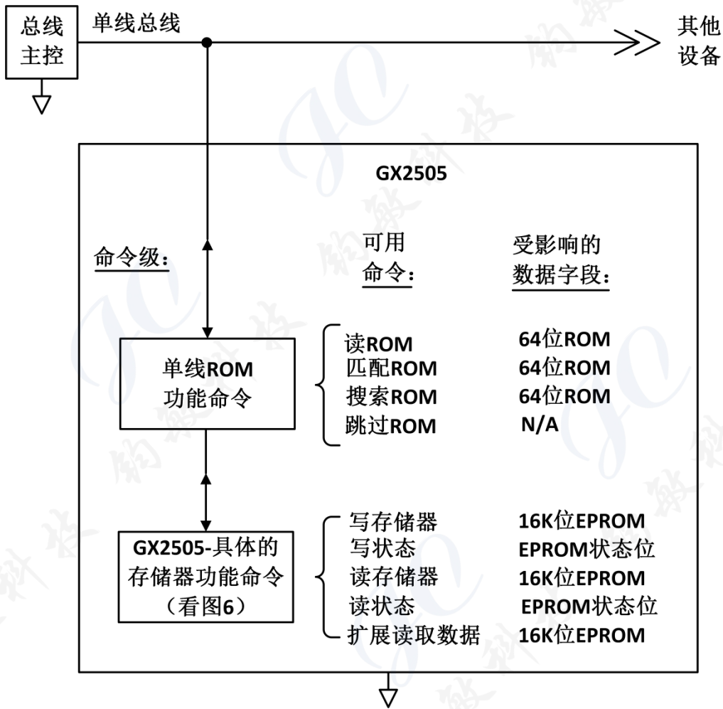
1-Wire 协议的层次结构 图 2
