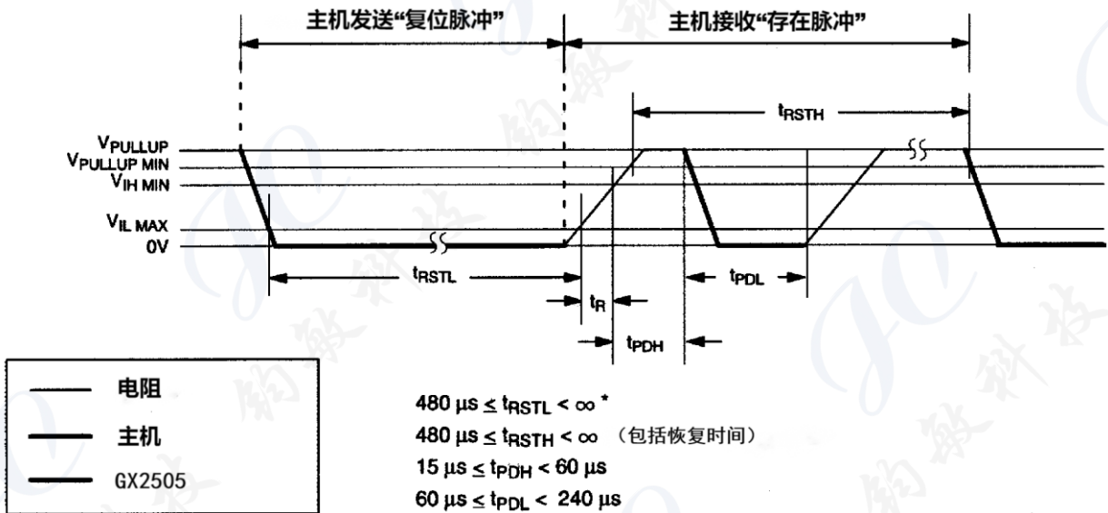
“复位和在线应答脉冲”的初始化时序 图9
