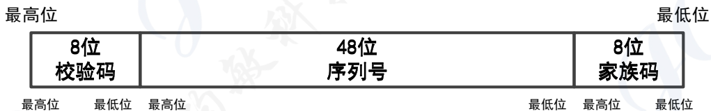
图 2 64 位 ROM ID
